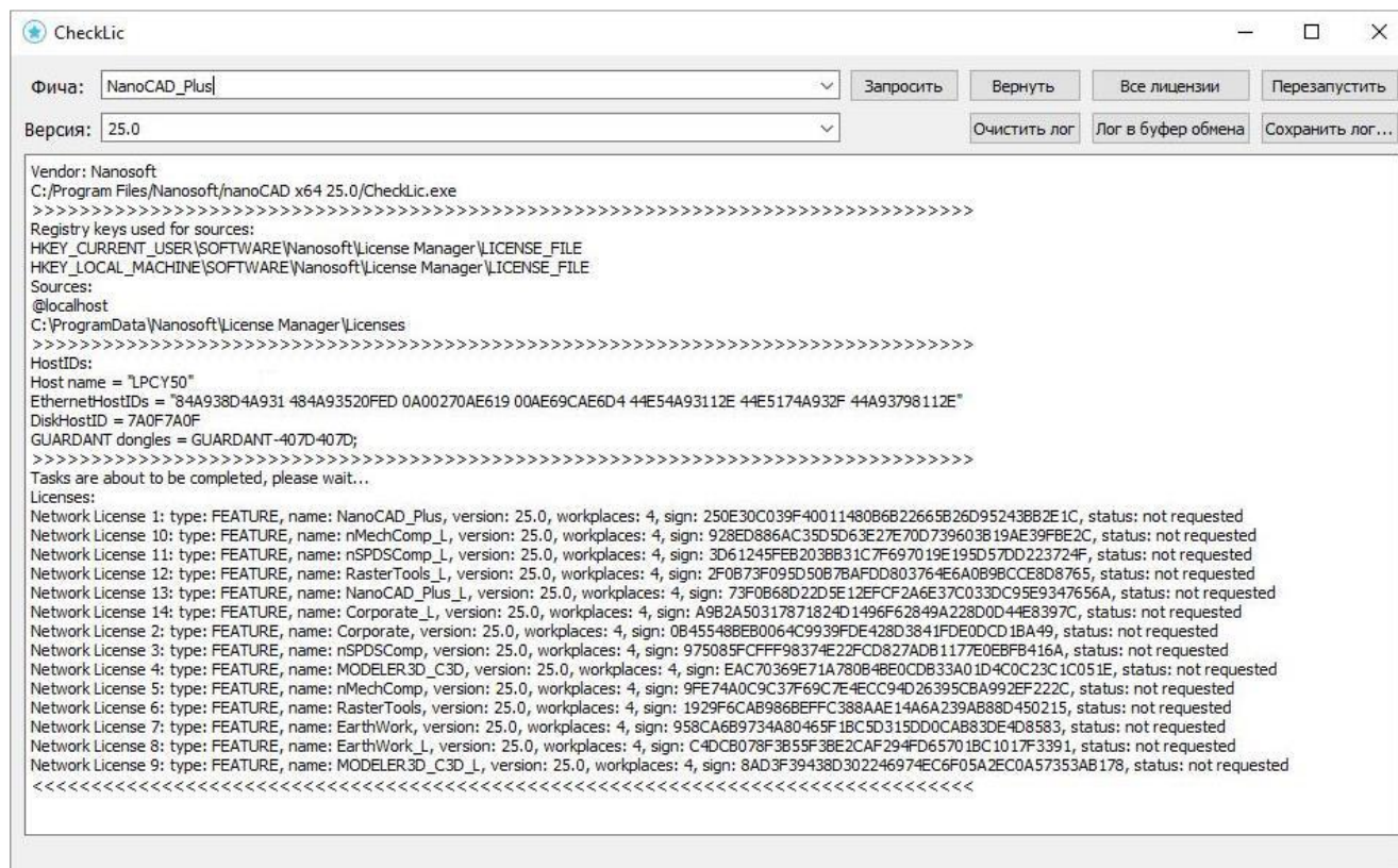
Утилита CheckLic
