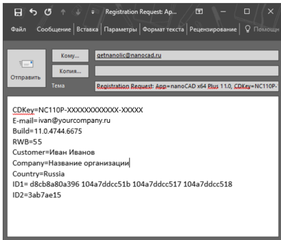
Электронное письмо с запросом лицензии
